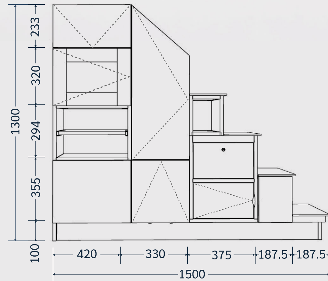
Vue Face
